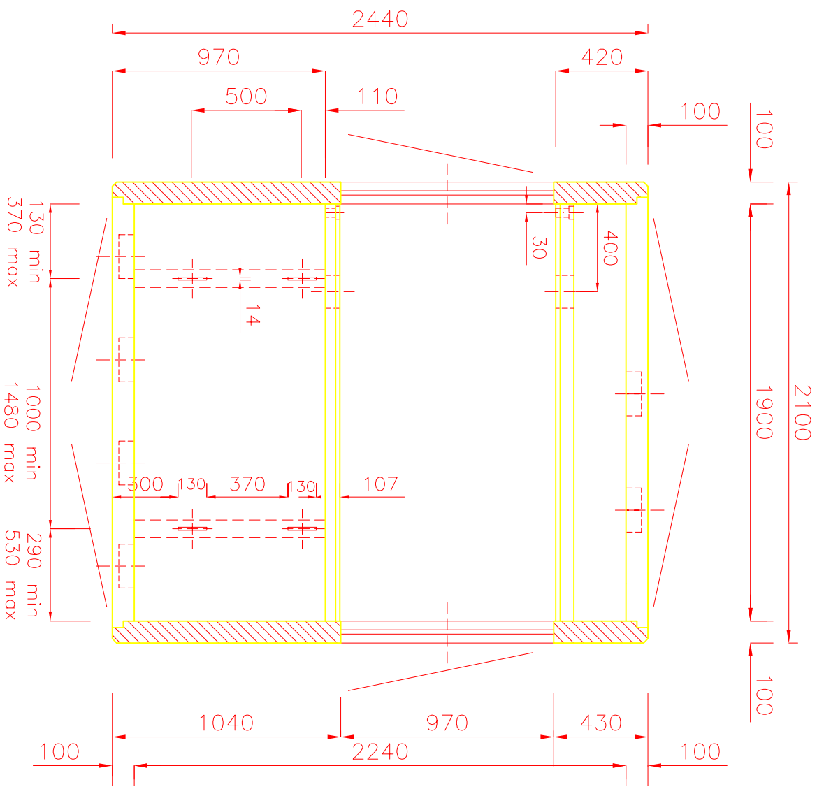
PIANTA BOX
