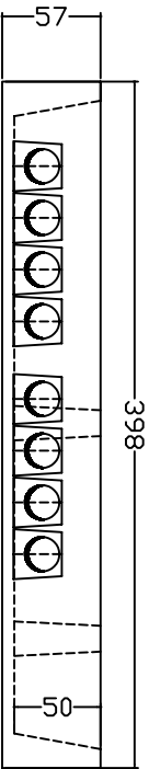
VISTA FRONTALE BASE A VASCA
