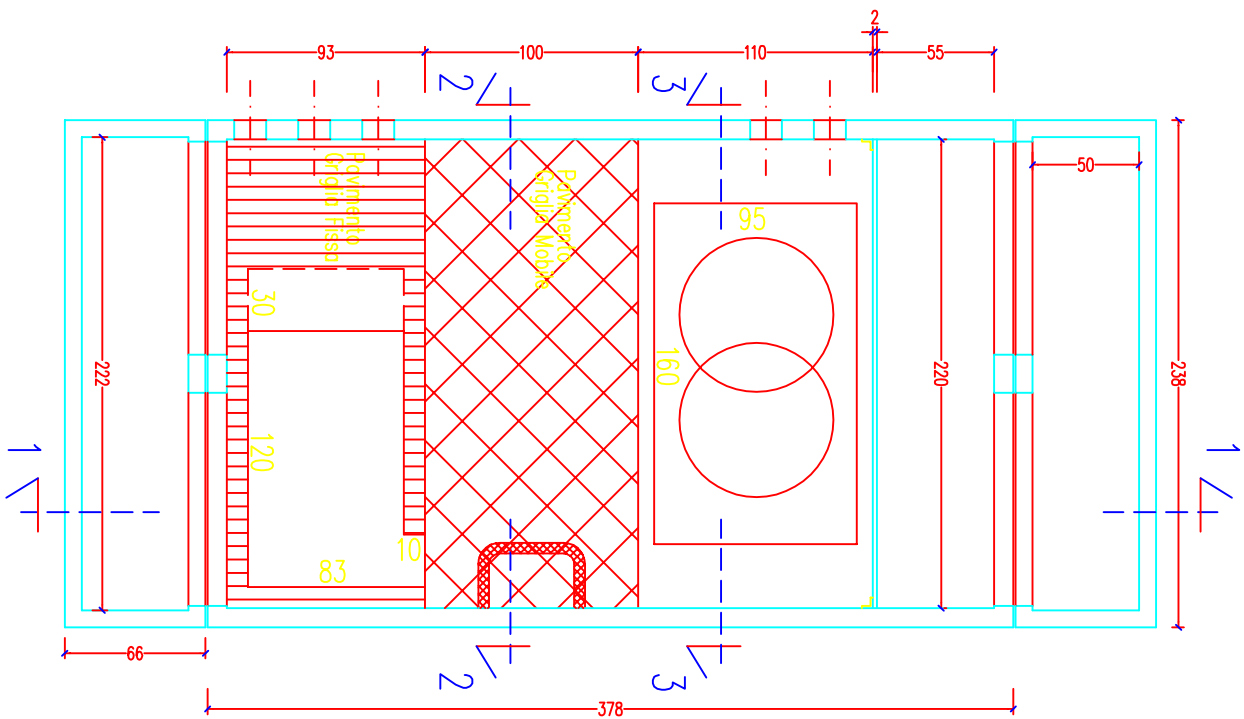
PIANTA CABINA
