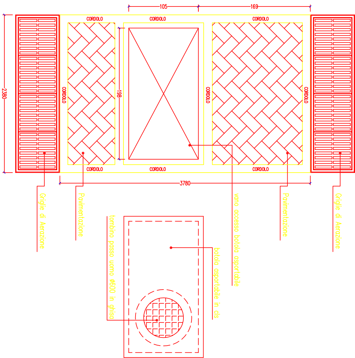
PIANTA COPERTURA CABINA
